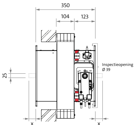
FD25 MF2 M
