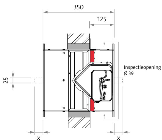
FD25 O R
